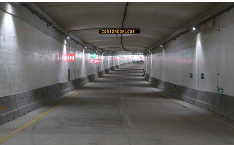
Túnel sumergido de Coatzacoalcos (México).
